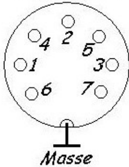
Ansicht Stecker (Lötseite)
